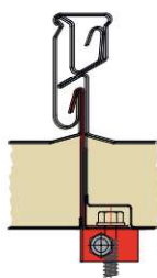
fixation supérieure
